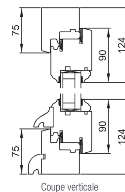
Coupe verticale
