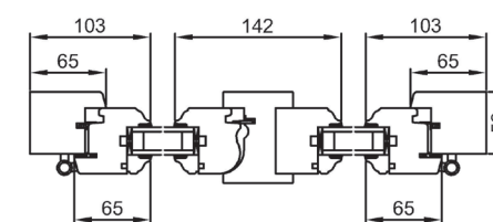
Coupe horizontale
