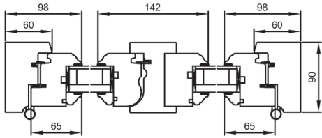
Coupe horizontale
