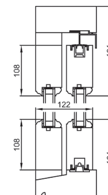
Coupe verticale
