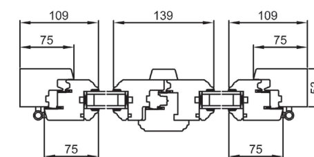
Coupe horizontale
