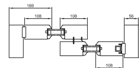
Coupe horizontale
