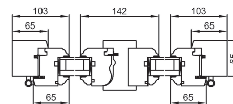
Coupe horizontale
