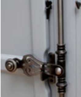
Usinage spécifique du montant du volet si fermeture par espagnolette
