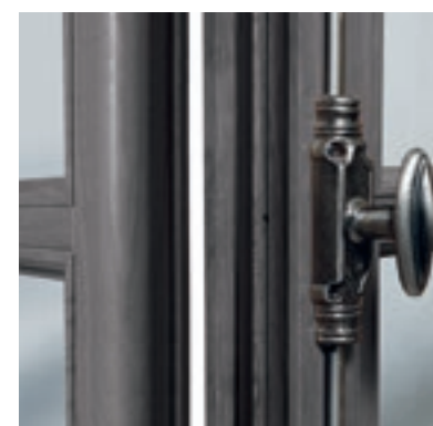
Fermeture à mouton et gueule de loup avec joint dans la gueule de loup
