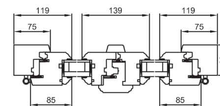
Coupe horizontale
