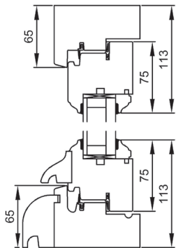
Coupe verticale
