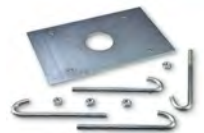
SIA2 Base d'ancrage avec agrafes pour WIDEL.
