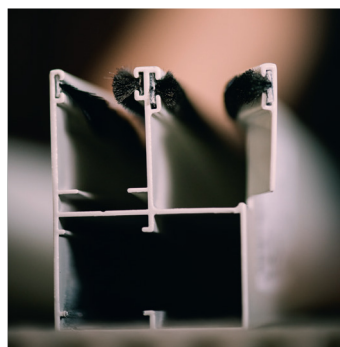
Zoom coulisse de la moustiquaire
