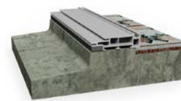
SEUIL ALU 20 mm . compatible PMR
